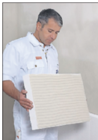
Multipor isoleringspladen monteres uden brug af dybler men udelukkende med Isochaux mørtlen, der også bruges til den efterfølgende pudning.
